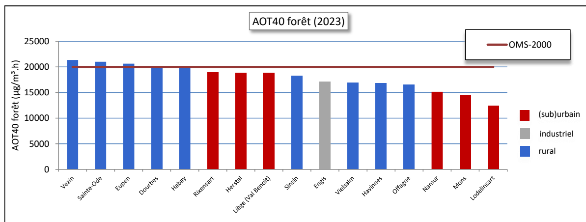
Figure 39 : AOT40 forêt - 2023
