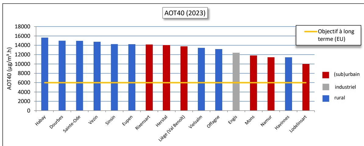
Figure 28 : AOT40 végétation – 2023
