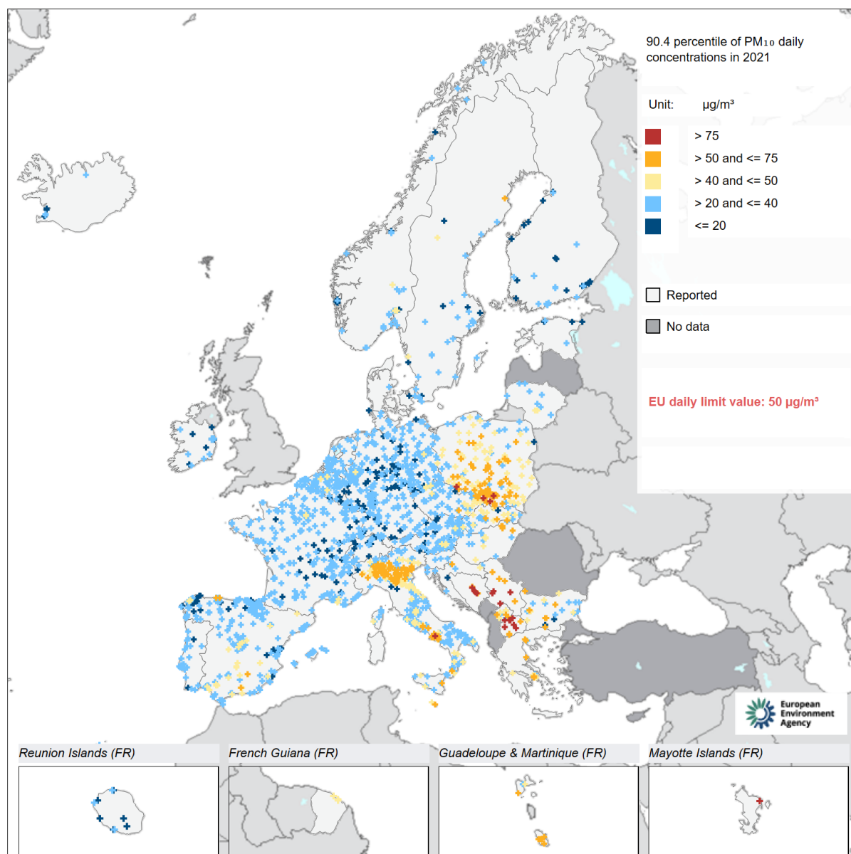
Figure 72 : Percentile 90.4 des moyennes journalières en PM10 (correspondant au 36 ème maximum) – Situation pour l’année 2021
