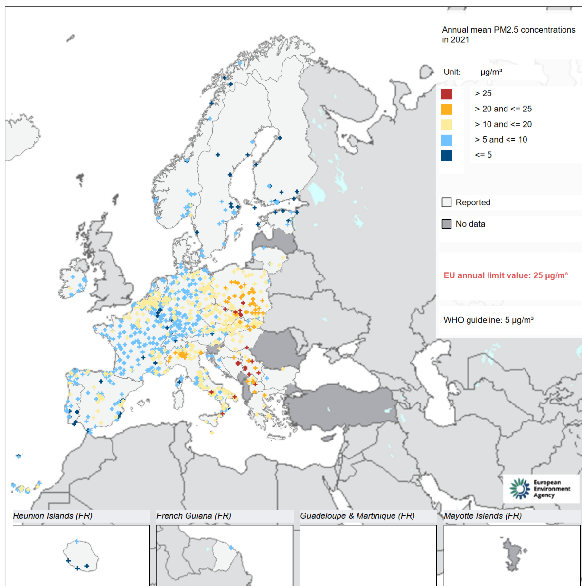
Figure 73 : Concentrations annuelles en PM 2.5 . Situation pour l'année 2021.
