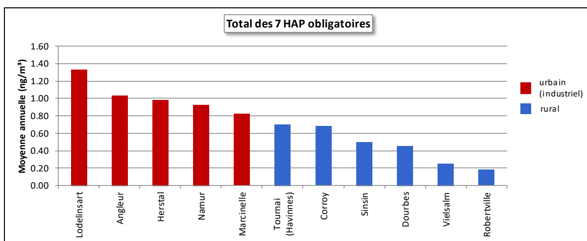
Figure 132 : Total des 7 HAP dont la mesure est obligatoire - Répartition des stations selon la moyenne annuelle en 2021
