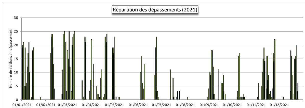
Figure 69 : Répartition des dépassements (PM2.5) en 2021
