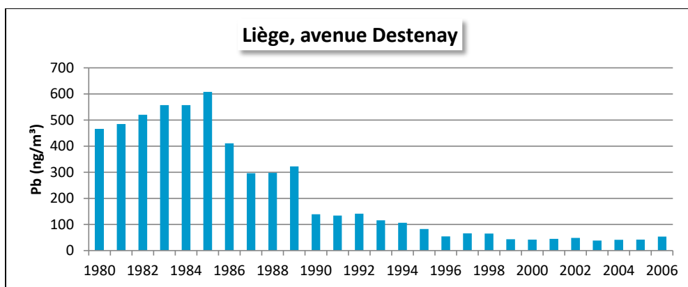
Figure 120 : Évolution à long terme des concentrations en plomb (mesure sur le total des particules en suspension - TSP) - Station de Liège, avenue Desténay
