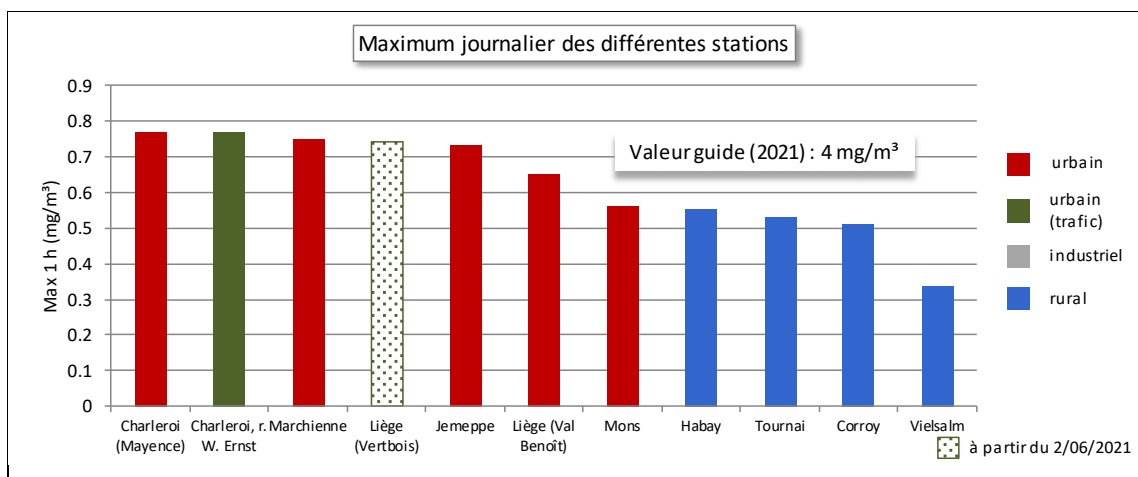
Figure 106 : Classement des stations en fonction des maxima horaires et journaliers en 2021
