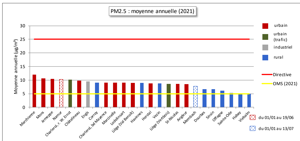
Figure 61 : Comparaison des moyennes annuelles de 2021 avec la valeur limite européenne et la valeur guide OMS (2021)
