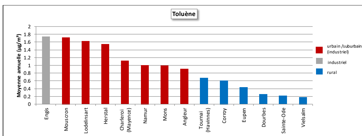
Figure 129 : Toluène - Répartition des stations selon la moyenne annuelle en 2021
