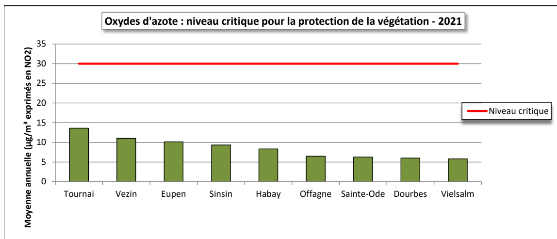
Figure 22 : Moyenne annuelle en oxydes d'azote et niveau critique pour la protection de la végétation - 2021
