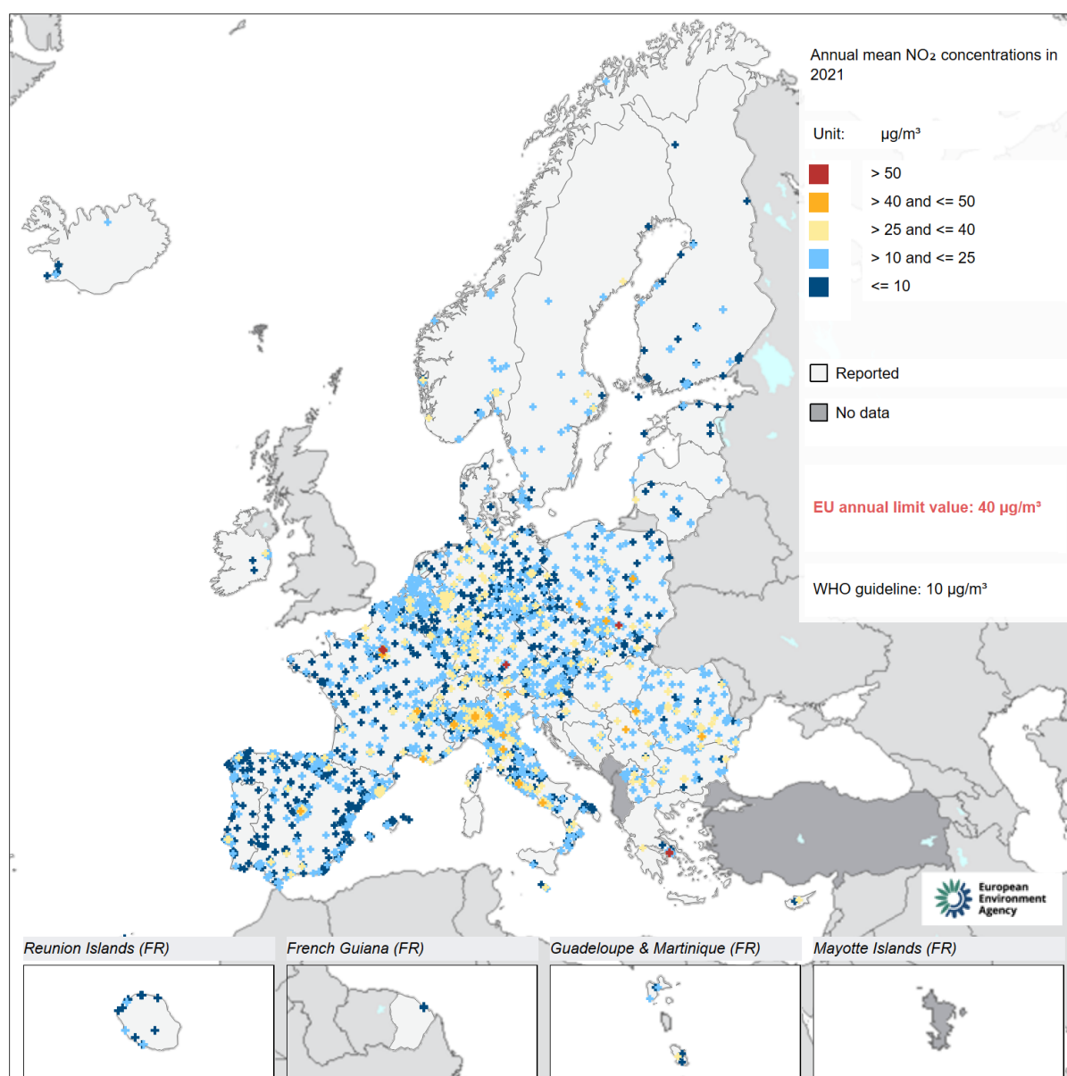
Figure 80 : Moyenne annuelle des concentrations de NO 2 (µg/m³) pour l'année 2021
