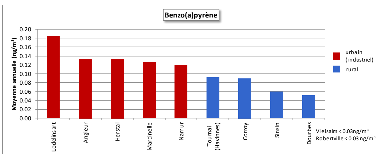
Figure 133 : Benzo(a)pyrène - Répartition des stations selon la moyenne annuelle en 2021
