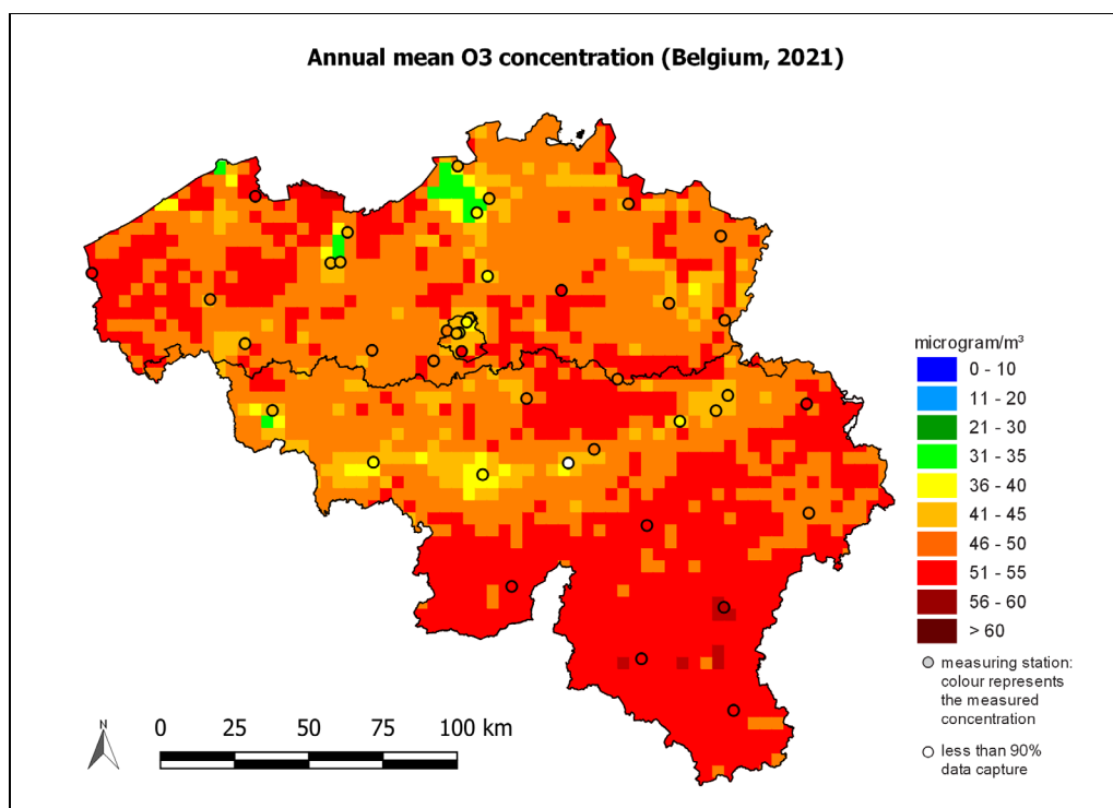
Figure 88 : Distribution spatiale de la concentration moyenne annuelle d'ozone en Belgique en 2021. Toutes les données ont été calculées sur base de la technique d'interpolation RIO.
