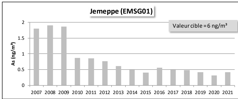
Figure 110 : Arsenic - Évolution des moyennes annuelles à Namur et Jemeppe
