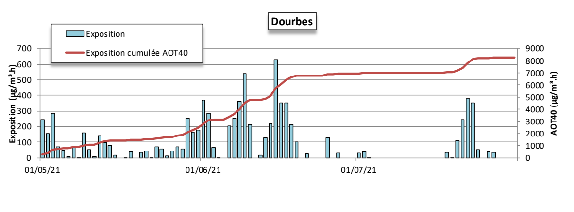
Figure 33 : Répartition de l'exposition - Station de Dourbes - 2021
