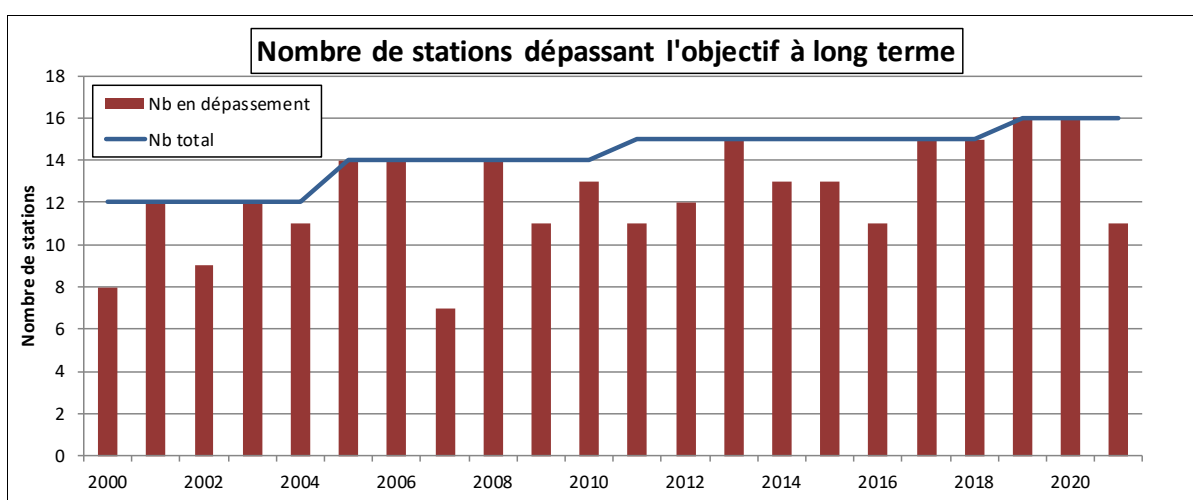
Figure 32 : Évolution du nombre de stations ne répondant pas à l'objectif à long terme
