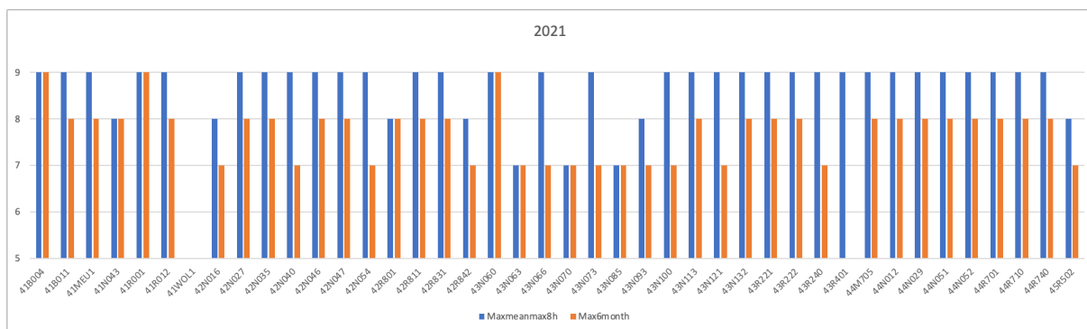
Figure 91 : Comparaison des périodes pour le maximum de la moyenne glissante sur 6 mois et du maximum de la moyenne glissante sur 6 mois des max 8h journaliers pour l'ensemble des stations de mesure, année 2021
