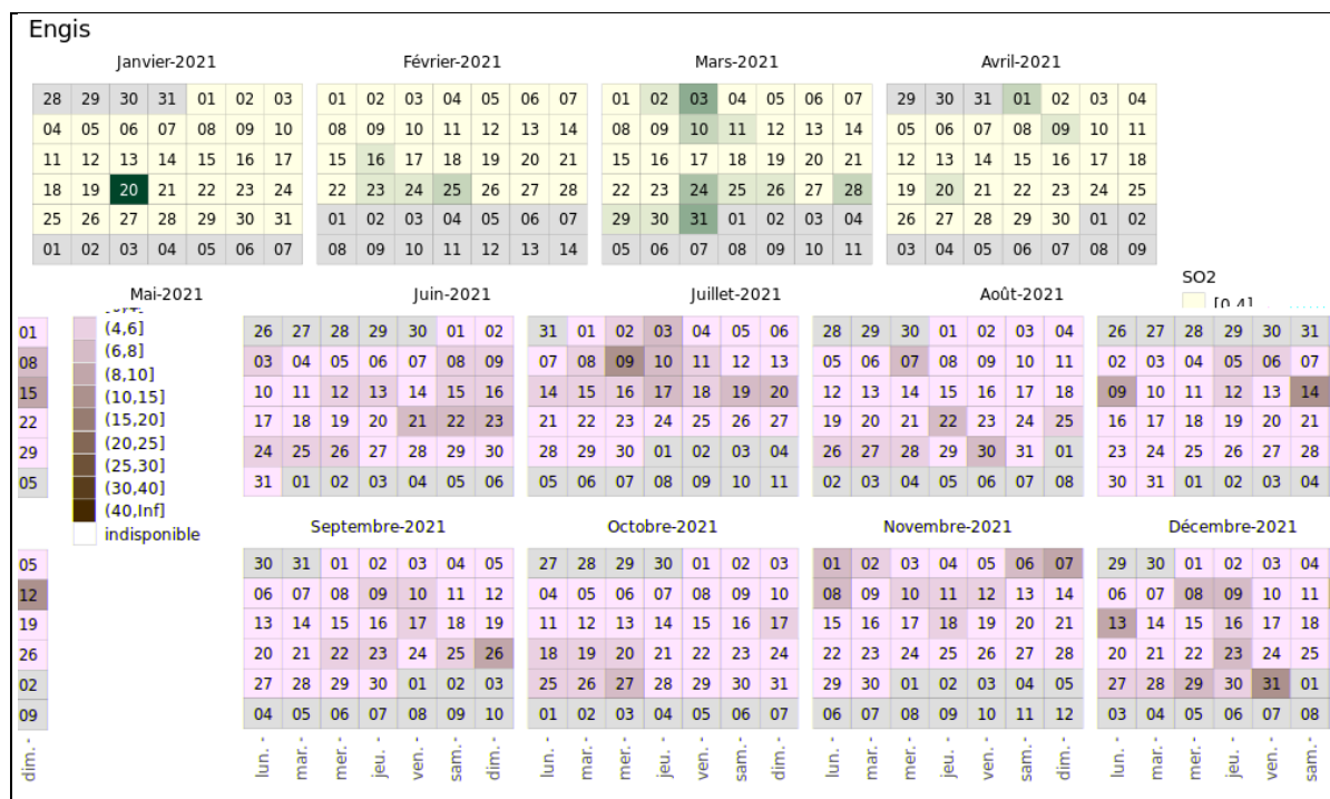
Figure 101 : Répartition au cours de l'année des moyennes journalières en dioxyde de soufre – Station d'Engis
