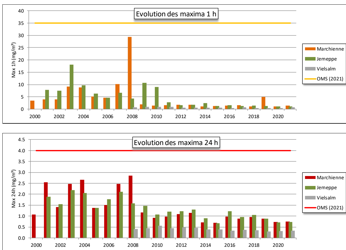
Figure 107 : Évolution à long terme des maxima horaires et journaliers - Stations de Marchienne, Jemeppe et Vielsalm
