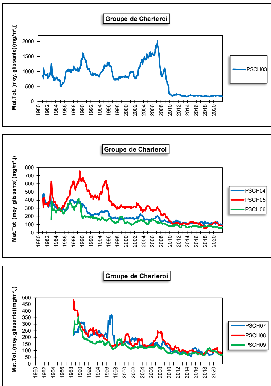
Figure 168 : Groupe de Charleroi - Évolution à long terme des retombées totales
