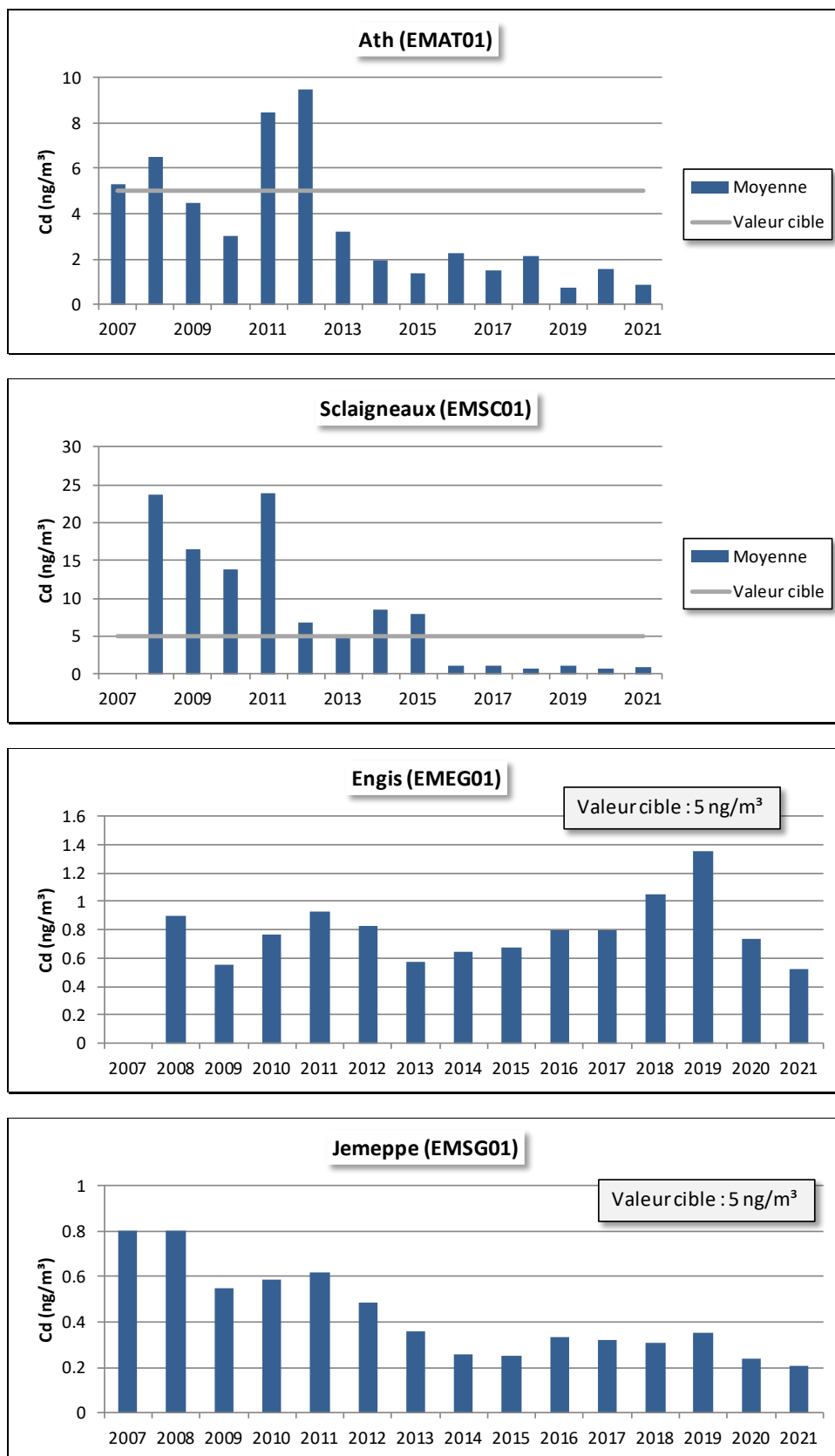
Figure 112 : Cadmium - Évolution des moyennes annuelles à Ath, Sclaigneaux, Engis et Jemeppe
