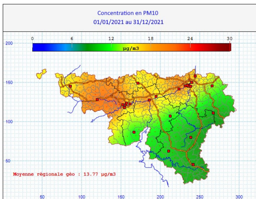
Figure 58 : Répartition des concentrations moyennes en particules PM10 - 2021 (interpolation par krigeage)
