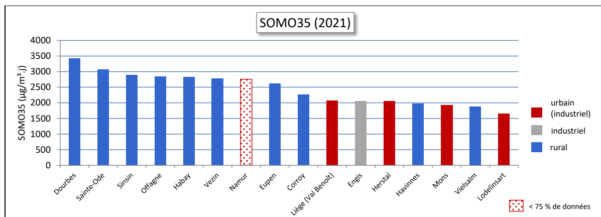
Figure 39 : Indicateur santé SOMO35 – 2021
