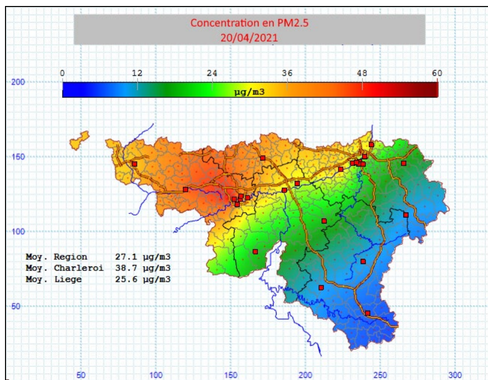
Figure 70 : Répartition spatiale des concentrations en PM2.5 – 20/04/2021
