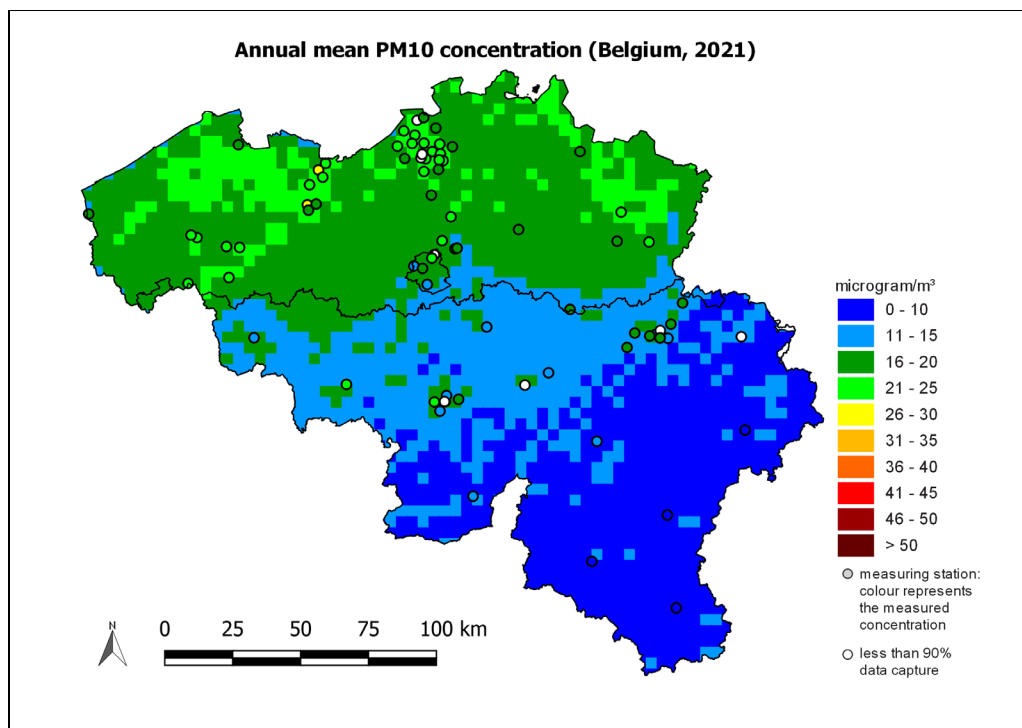
Figure 74 : Moyenne annuelle des concentrations de PM10 ( \mu\text{g}/\text{m}^3 ) pour 2021. Toutes les données ont été calculées sur base de la technique d'interpolation RIO.
