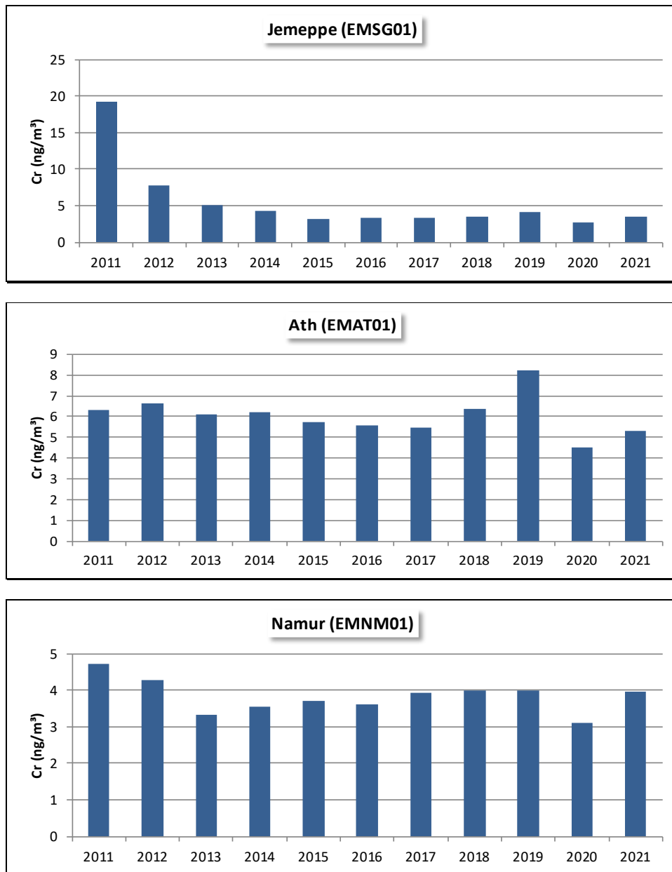
Figure 114 : Chrome - Évolution des moyennes annuelles à Jemeppe, Ath et Namur
