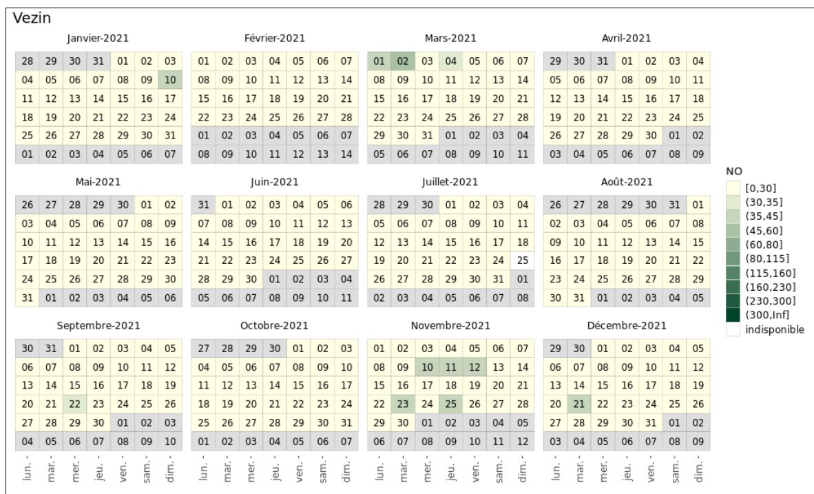
Figure 24 : Monoxyde d'azote - Répartition au cours de l'année des maxima horaires - Stations de Charleroi, bd Mayence, Herstal et Vezin
