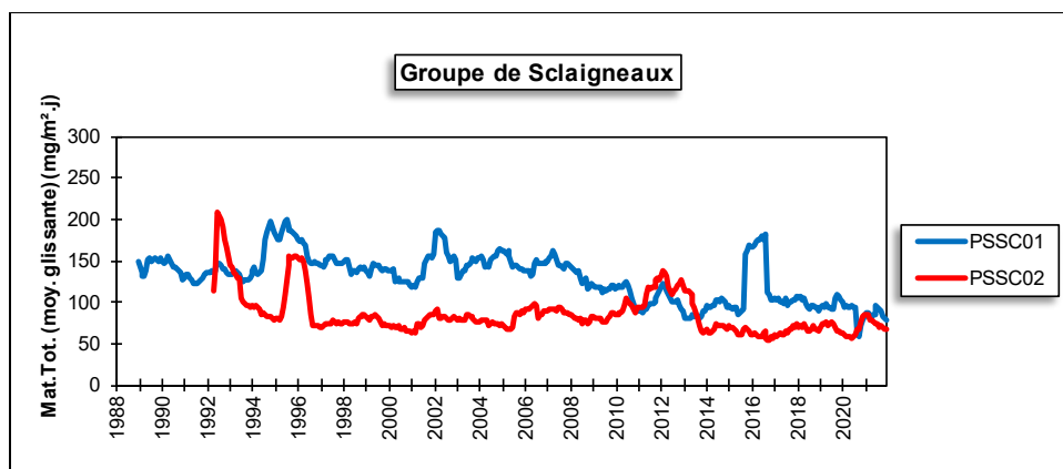
Figure 191 : Groupe de Sclaigheaux - Évolution à long terme des retombées totales
