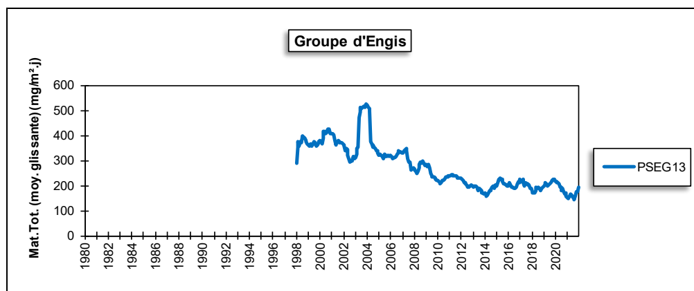
Figure 203 : Groupe d'Engis - Évolution à long terme des retombées totales
