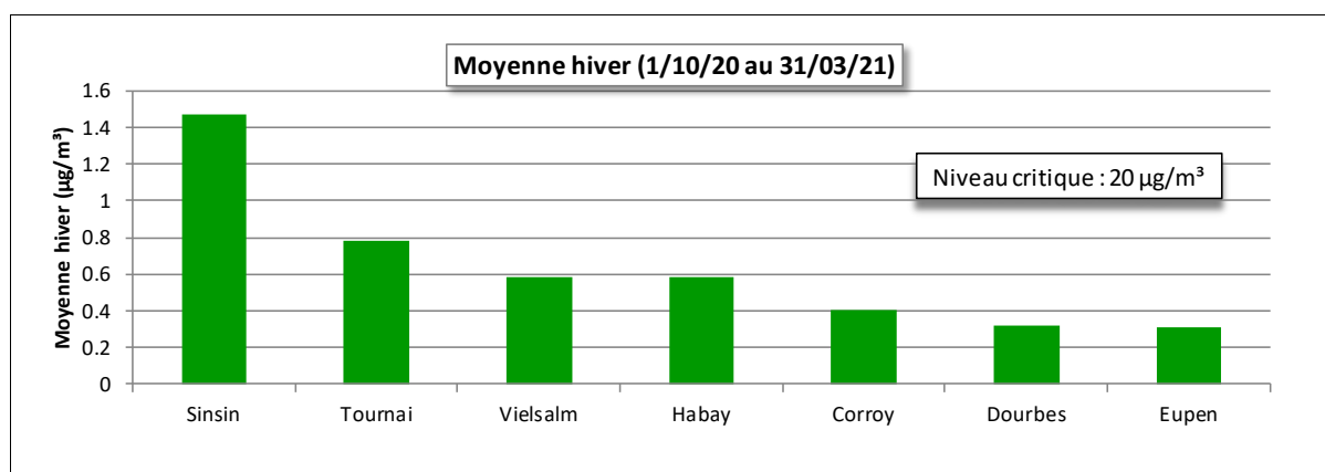
Figure 98 : Moyennes hivernales 2020-2021
