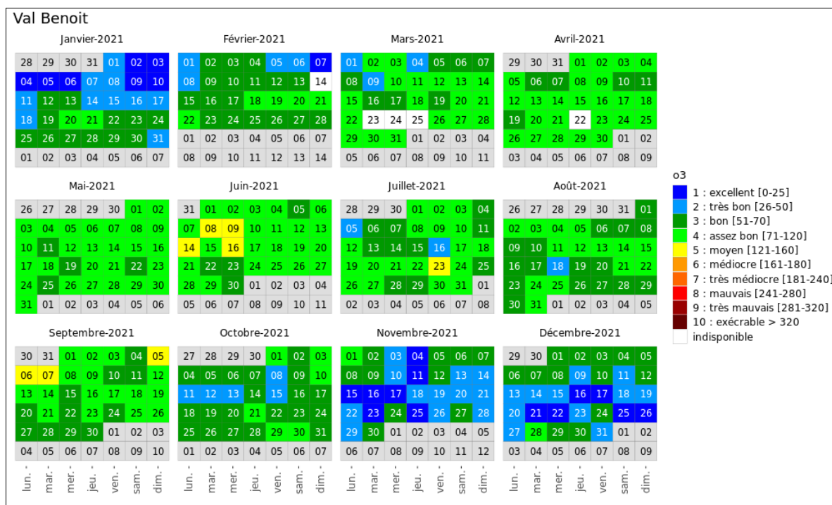
Figure 44 : Ozone - Répartition au cours de l'année de l'indice BelAQI - Stations de Corroy, Sainte-Ode et Liège (Val-Benoît)
