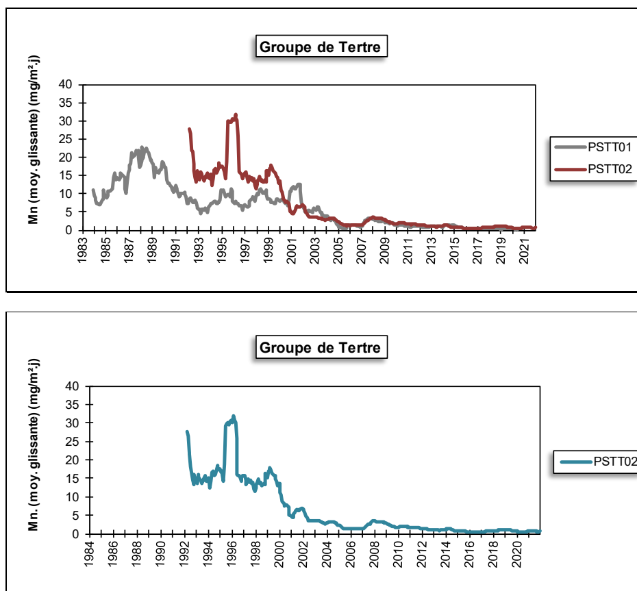
Figure 155 : Groupe de Tertre - Évolution à long terme des retombées en manganèse
