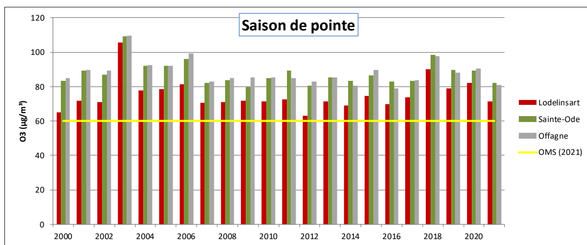
Figure 38 : Évolution à long terme de la moyenne pour la saison de pointe - Stations de Lodelinsart, Sainte-Ode et Offagne
