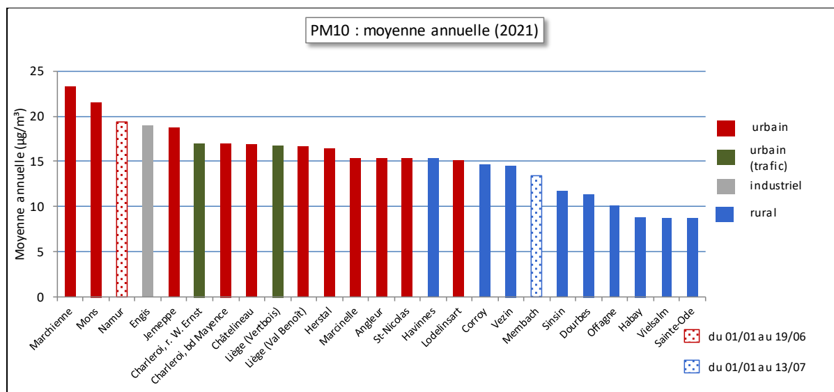
Figure 45 : PM10 - Répartition des stations selon la moyenne annuelle en 2021
