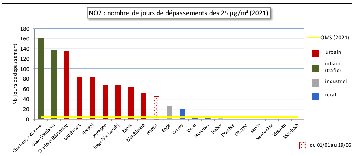
Figure 17 : Dioxyde d'azote - Classement des stations en fonction du nombre de dépassements journaliers – 2021
