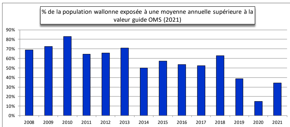
Figure 57 : Estimation de la proportion de la population wallonne exposée à une concentration supérieure à la recommandation OMS-2021 (15 µg/m³/an)
