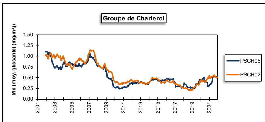
Figure 167 : Jauges de Dampremy - Évolution à long terme des retombées en manganèse
