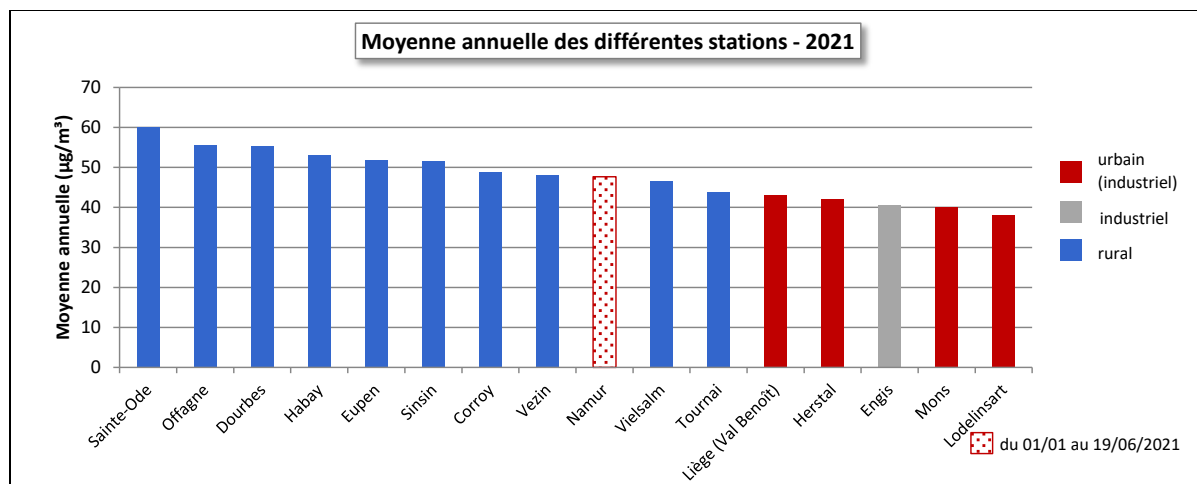
Figure 25 : Ozone - Répartition des stations selon la moyenne annuelle en 2021
