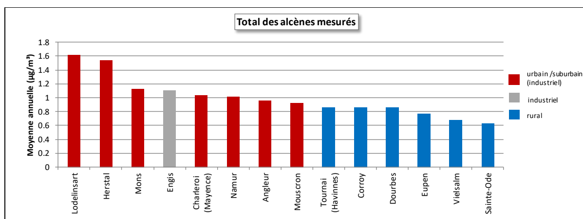
Figure 126 : Total des alcènes mesurés - Répartition des stations selon la moyenne annuelle en 2021
