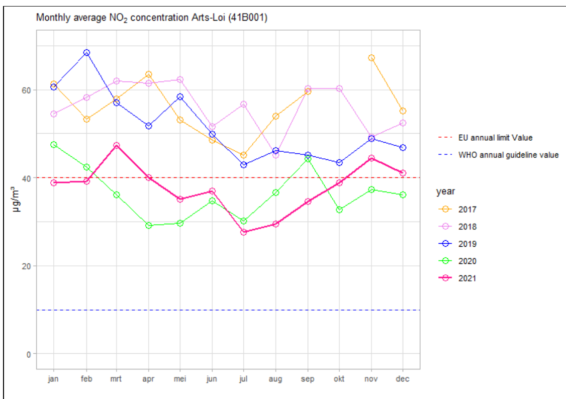
Figure 82 : Concentrations moyennes mensuelles de NO 2 (période 2017-2021) carrefour Arts-Loi (site de mesure 41B001)
