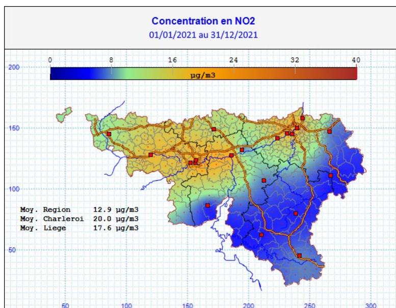
Figure 15 : Répartition géographique des moyennes annuelles
