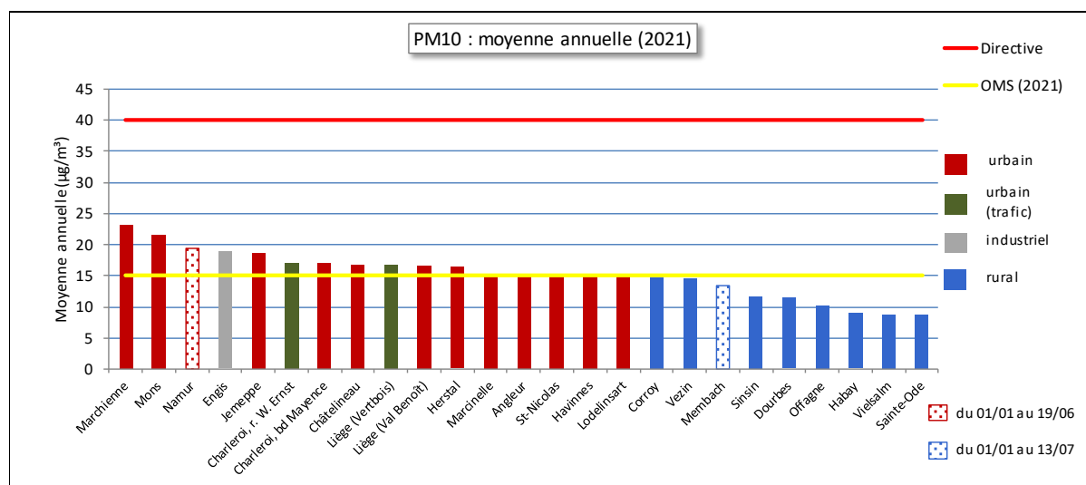
Figure 54 : Comparaison des moyennes annuelles de 2021 avec la valeur limite européenne et la valeur guide OMS (2021)
