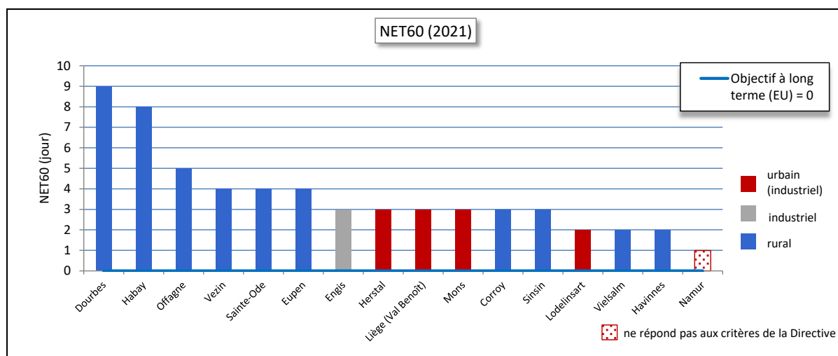
Figure 27 : Répartition des stations selon le NET60 pour 2021
