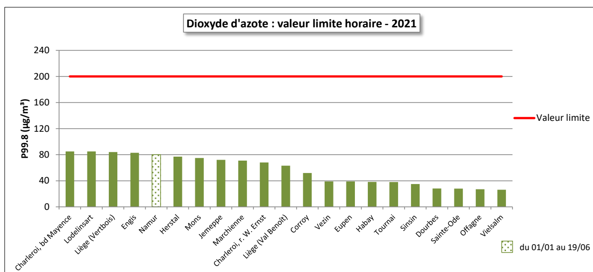
Figure 11 : Dioxyde d'azote – P99.8 et valeur limite horaire en 2021
