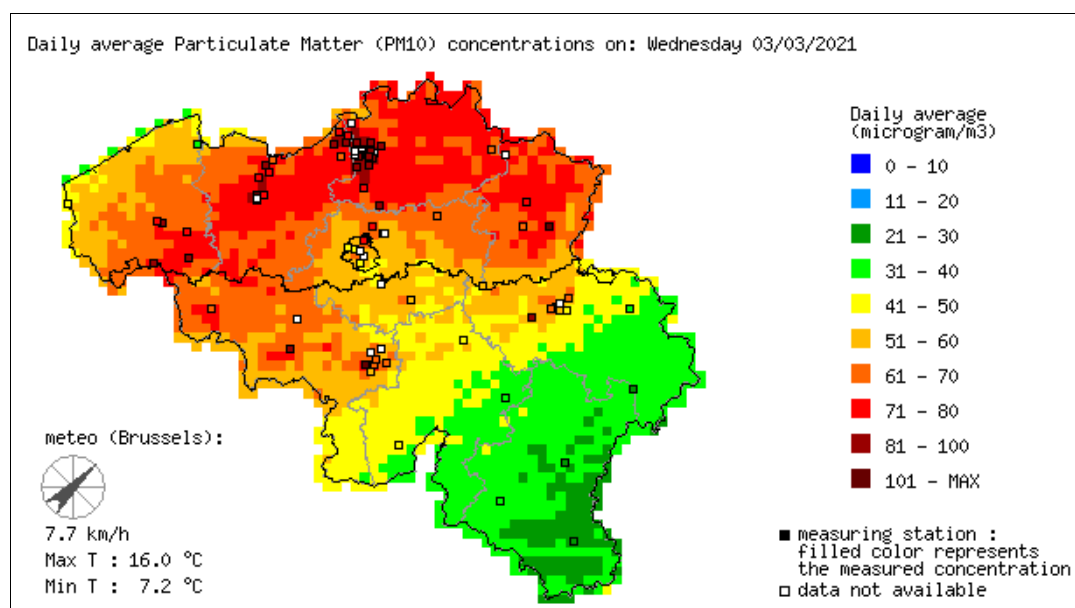
Figure 78 : 03/03/2021 - Moyenne journalière des concentrations de particules fines PM10 (méthode d'interpolation RIO)
