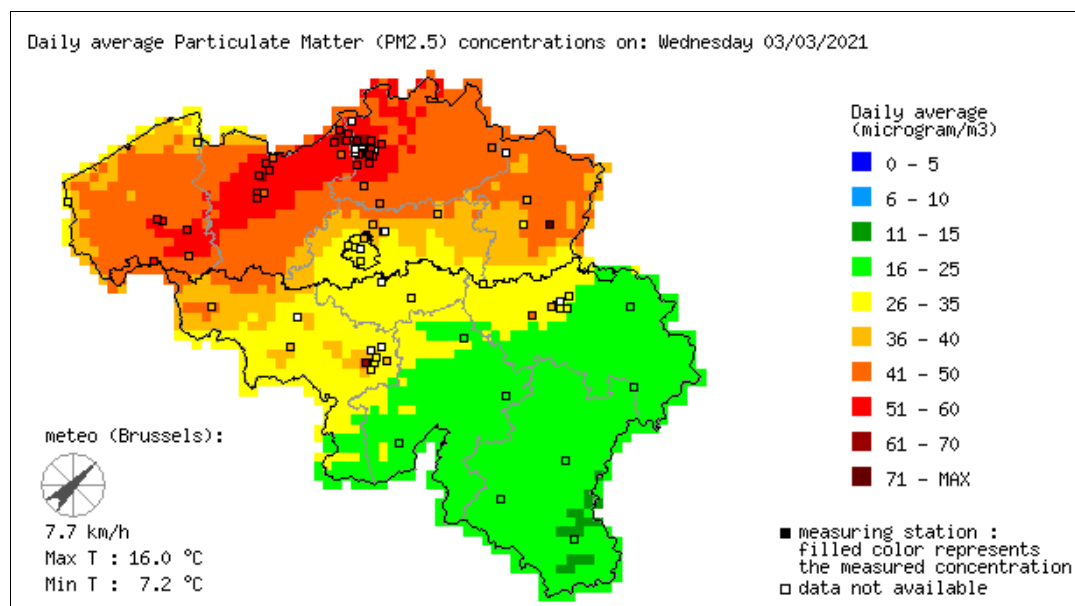
Figure 77 : 03/03/2021 - Moyenne journalière des concentrations de particules fines PM2.5 (méthode d'interpolation RIO)
