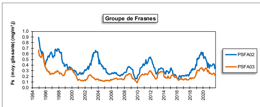
Figure 145 : Groupe de Frasnes-lez-Anvaing - Évolution à long terme des retombées en fluorures
