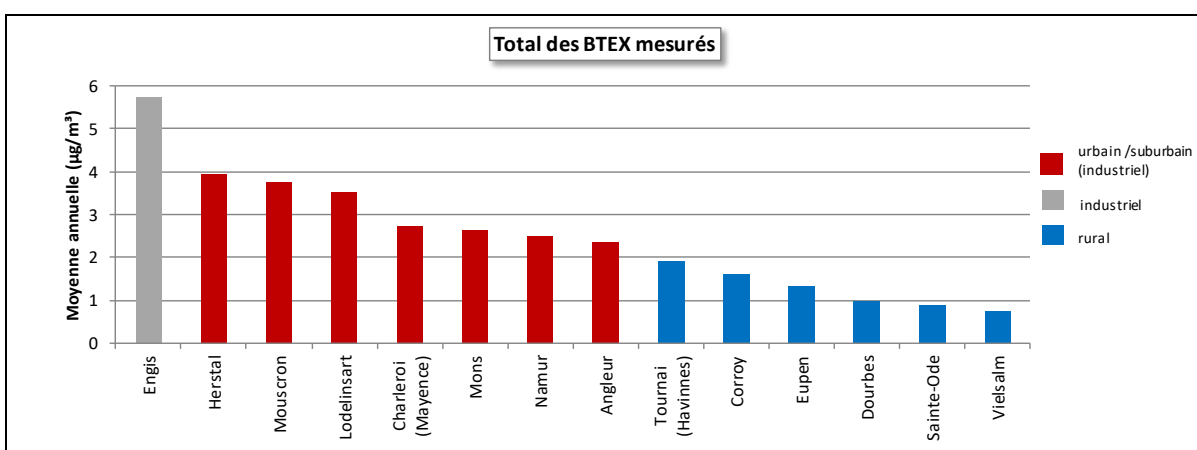
Figure 127 : Total des BTEX mesurés - Répartition des stations selon la moyenne annuelle en 2021
