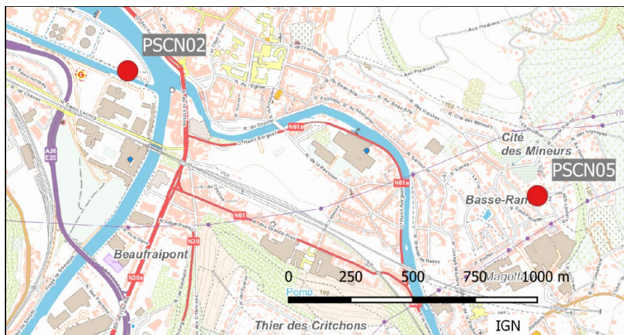
Figure 206 : Groupe de Chênée-Angleur - Localisation des stations
