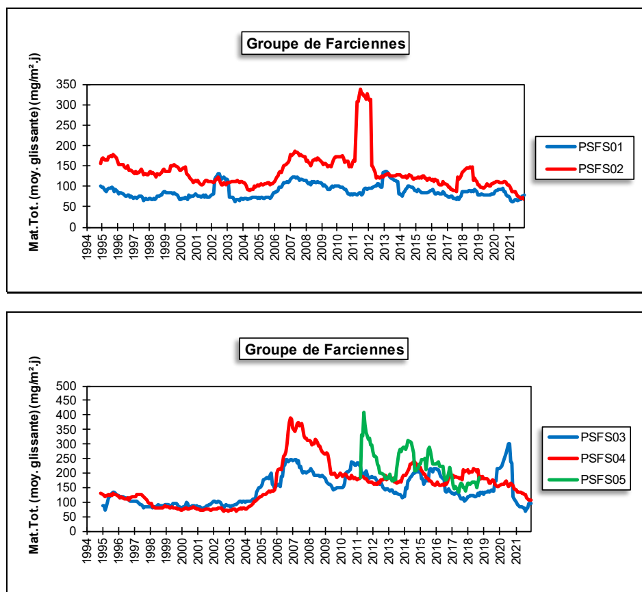
Figure 174 : Groupe de Farciennes - Évolution à long terme des retombées totales
