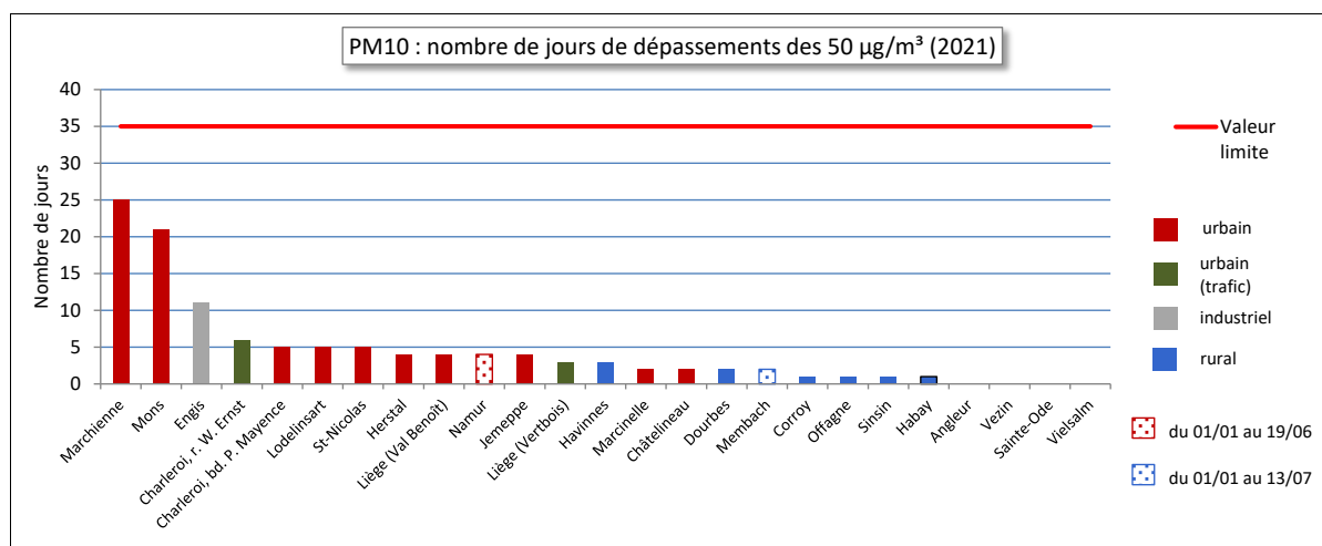
Figure 46 : PM10 - Classement des stations en fonction du nombre de dépassements journaliers (EU - 50 \mu\text{g}/\text{m}^3 ) – 2021
