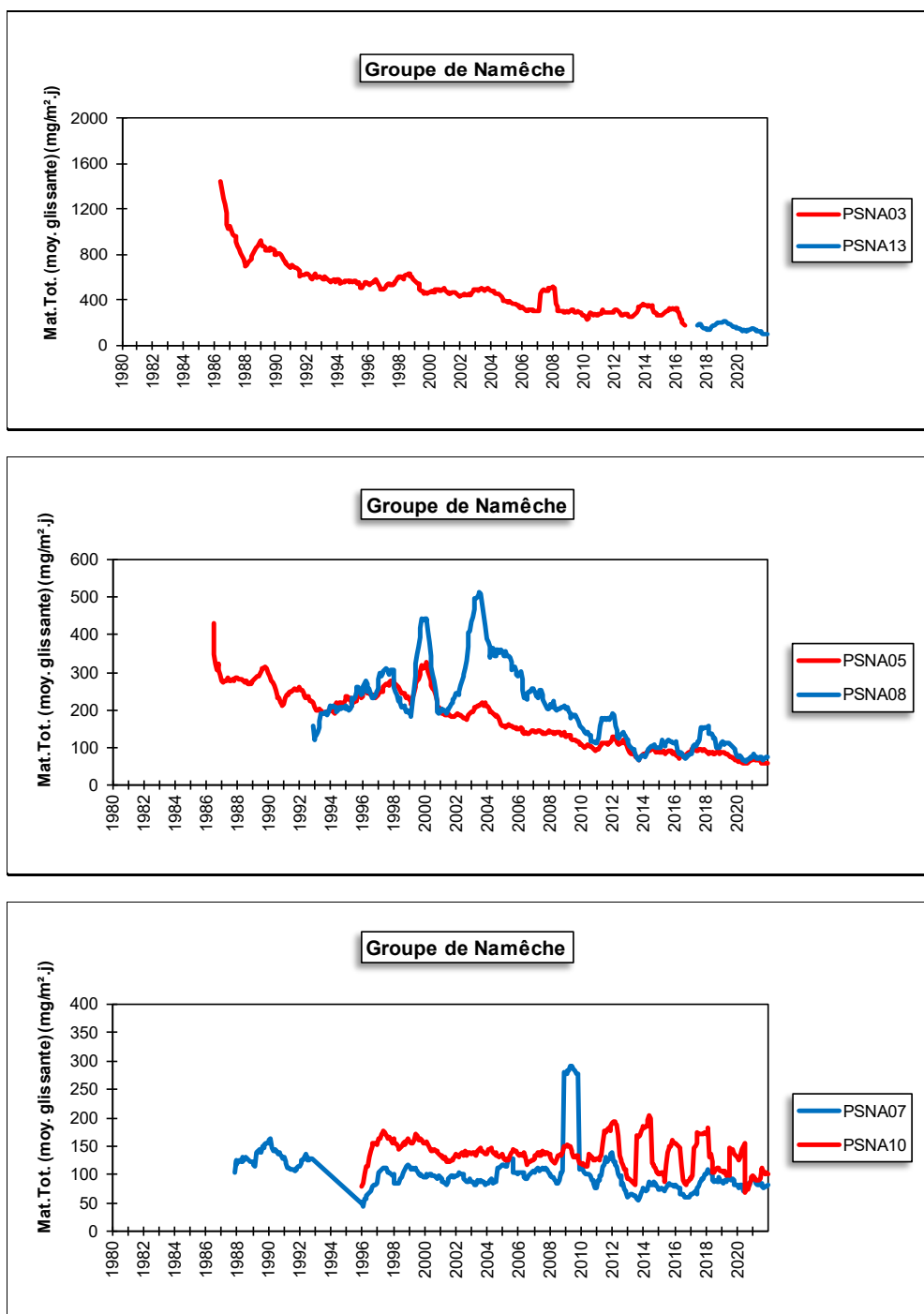
Figure 188 : Groupe de Namêche - Évolution à long terme des retombées totales
