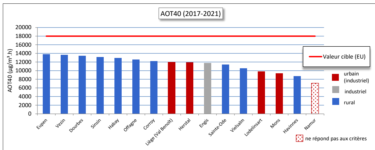
Figure 30 : AOT40 végétation - Moyenne 2017 à 2021
