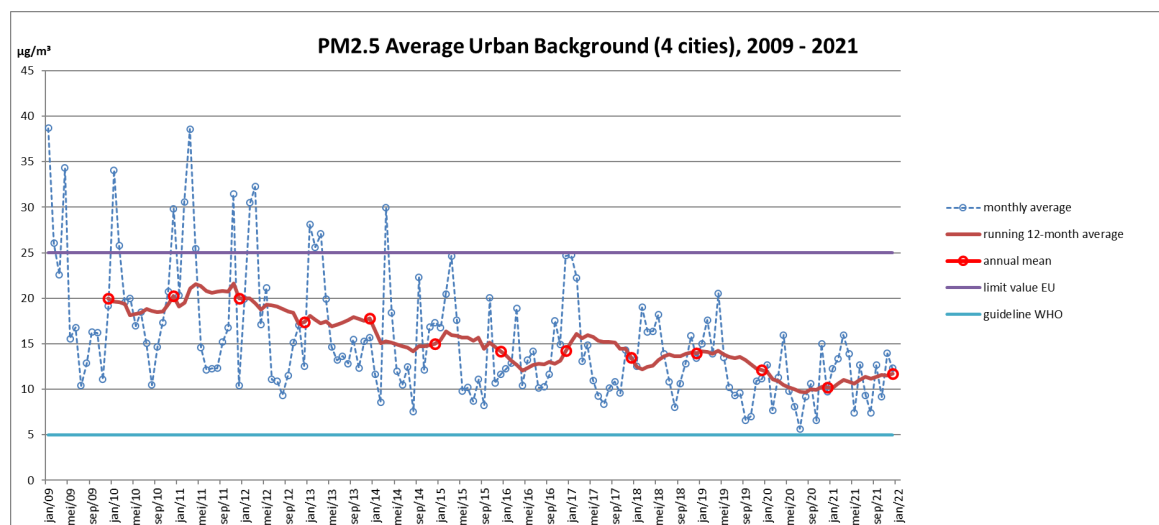
Figure 76 : Concentrations moyennes mensuelles entre 2009 et 2021 sur la base de mesures effectuées dans 4 sites de mesure de fond urbain (Gand, Anvers, Bruxelles et Charleroi).
