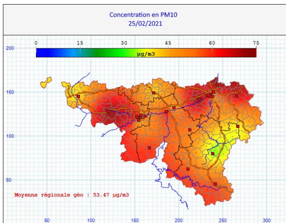
Figure 52 : Répartition spatiale des concentrations en PM10 – 25/02/2021
