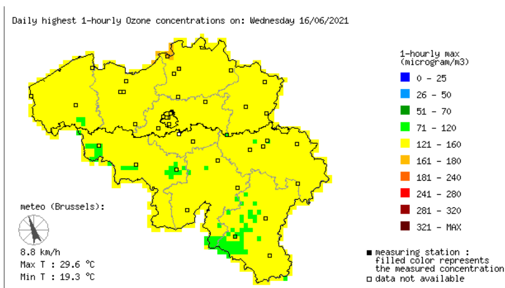
Figure 93 : Concentrations d'ozone horaires maximales du 16 juin 2021
