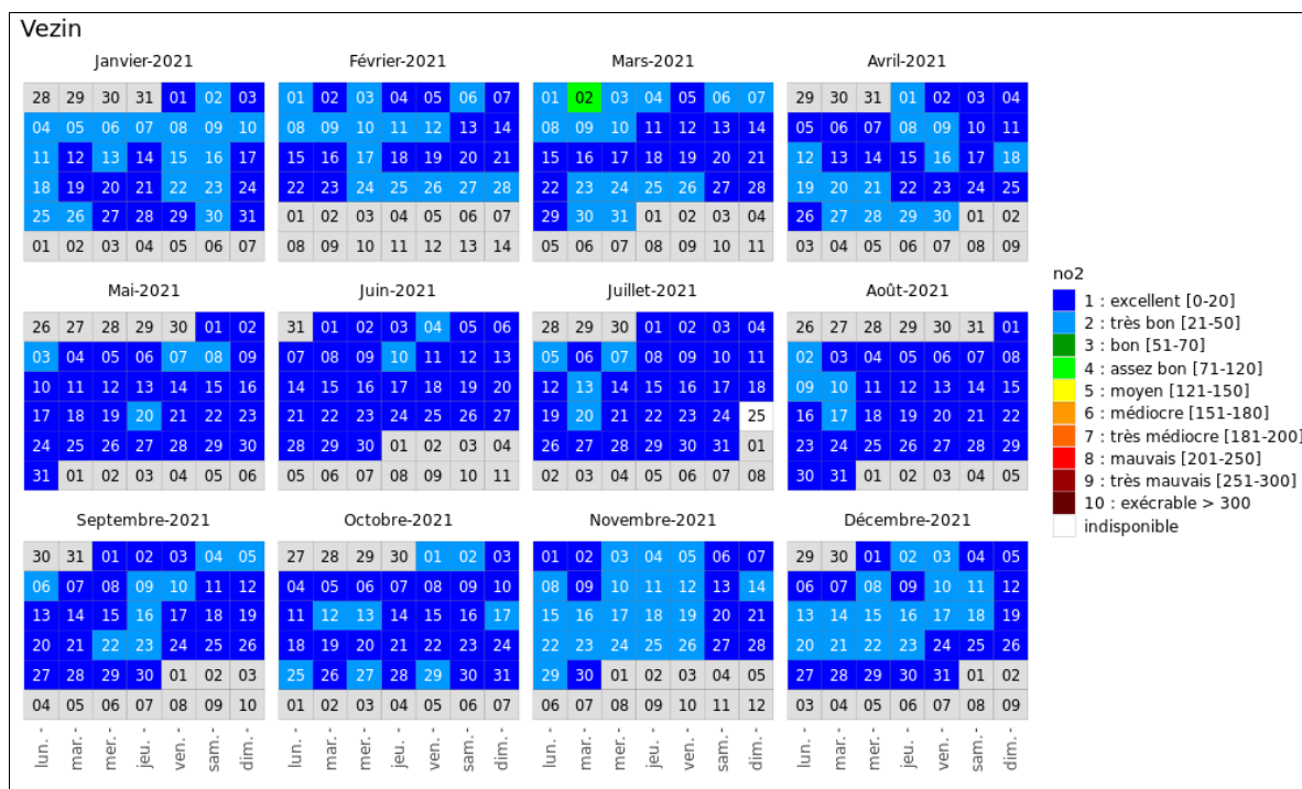
Figure 23 : Dioxyle d'azote - Répartition au cours de l'année de l'indice BelAQI - Stations de Charleroi, bd Mayence, Herstal et Vezin
