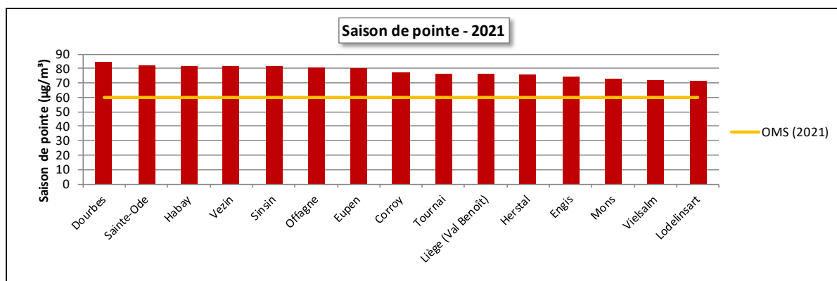
Figure 37 : Classement des stations en fonction de la moyenne pour la saison de pointe - 2021
