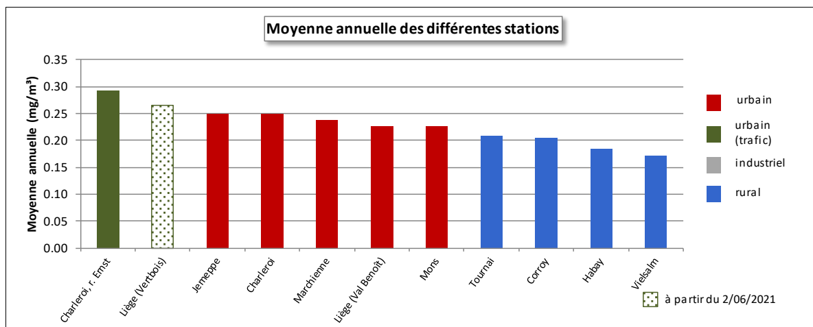
Figure 102 : Monoxyde de carbone – Répartition selon la moyenne annuelle en 2021
