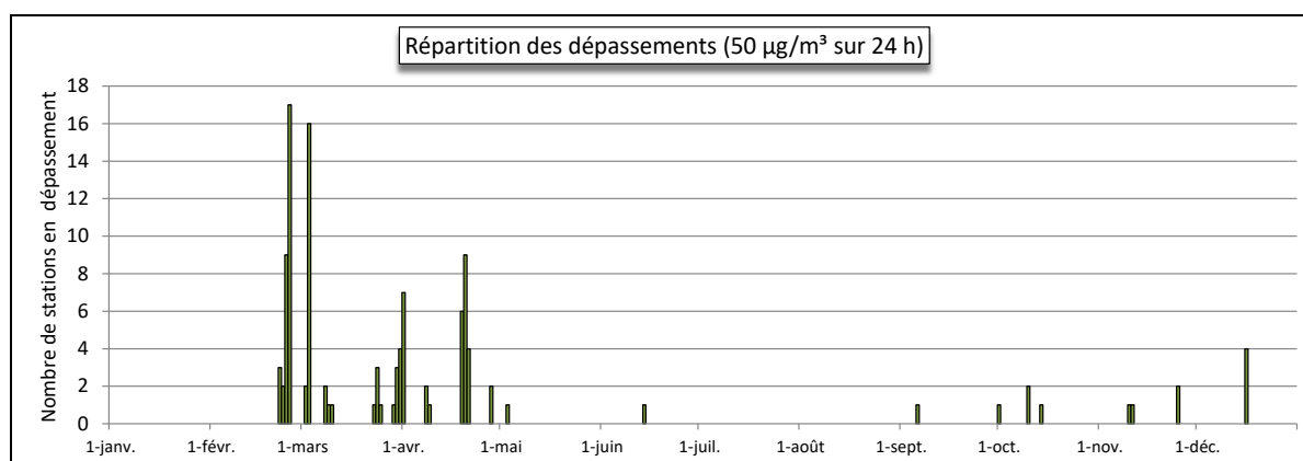
Figure 51 : Évolution temporelle du nombre de stations en dépassement de la norme journalière (EU) – 2021
