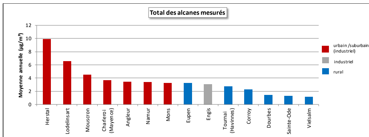
Figure 125 : Total des alcanes mesurés - Répartition des stations selon la moyenne annuelle en 2021
