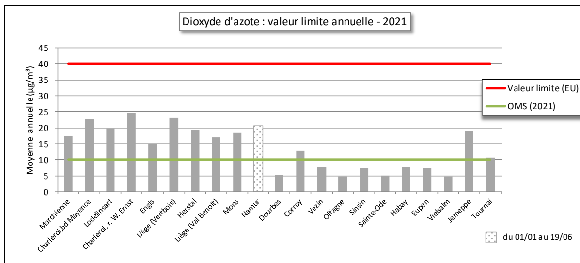
Figure 13 : Dioxyde d'azote – Valeur limite annuelle - 2021
