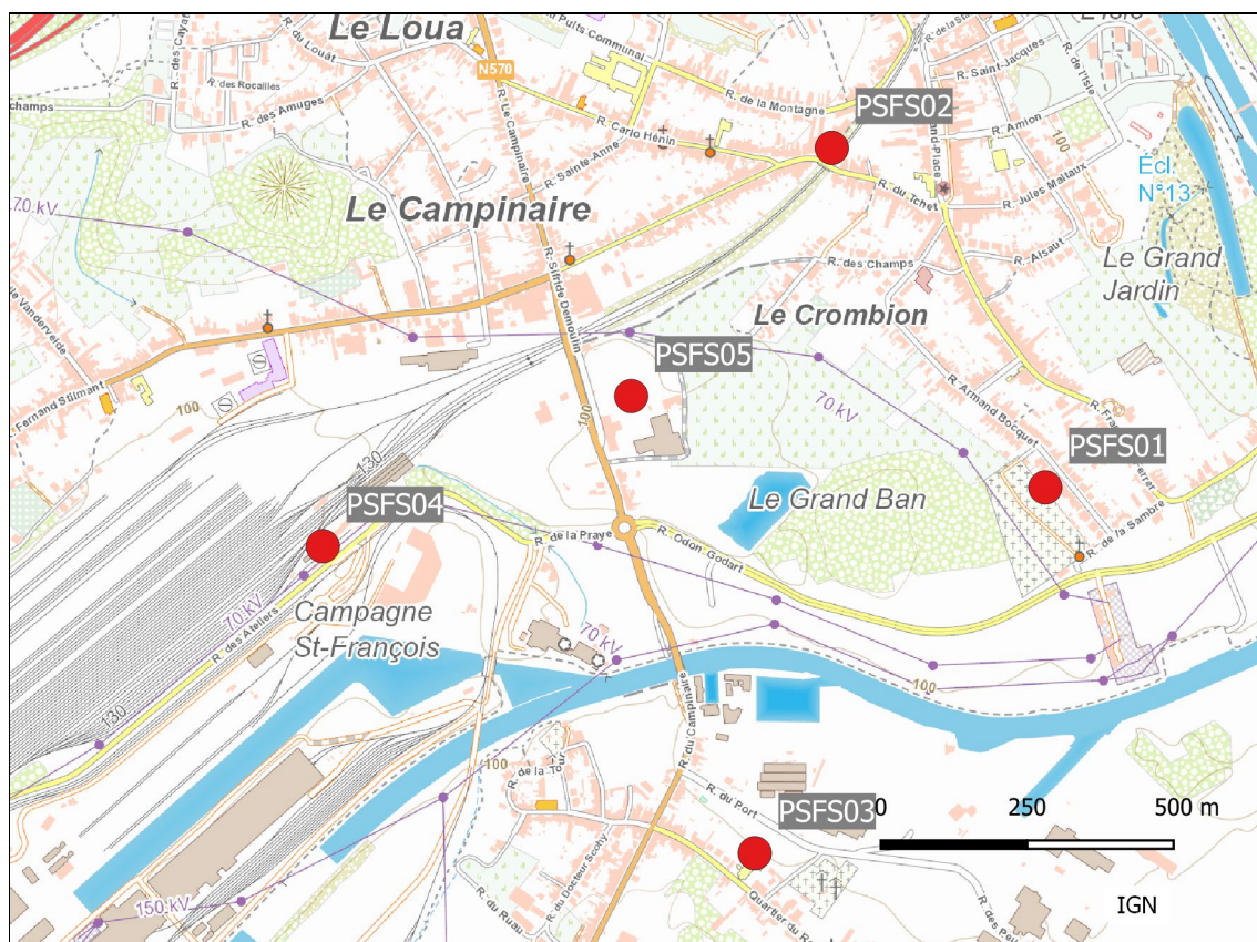
Figure 170 : Groupe de Farciennes - Localisation des stations
