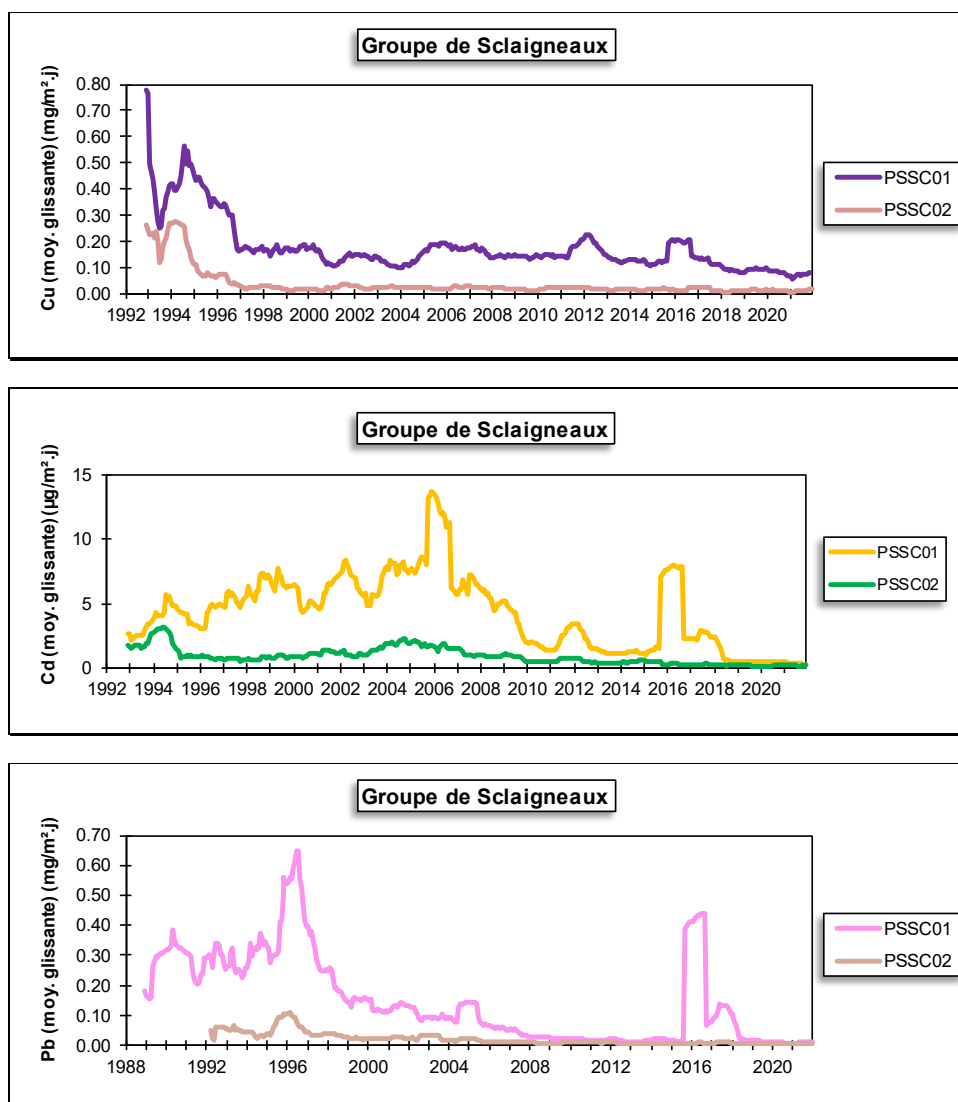
Figure 190 : Groupe de Sclaigheaux - Évolution à long terme des retombées en cuivre, cadmium et plomb
