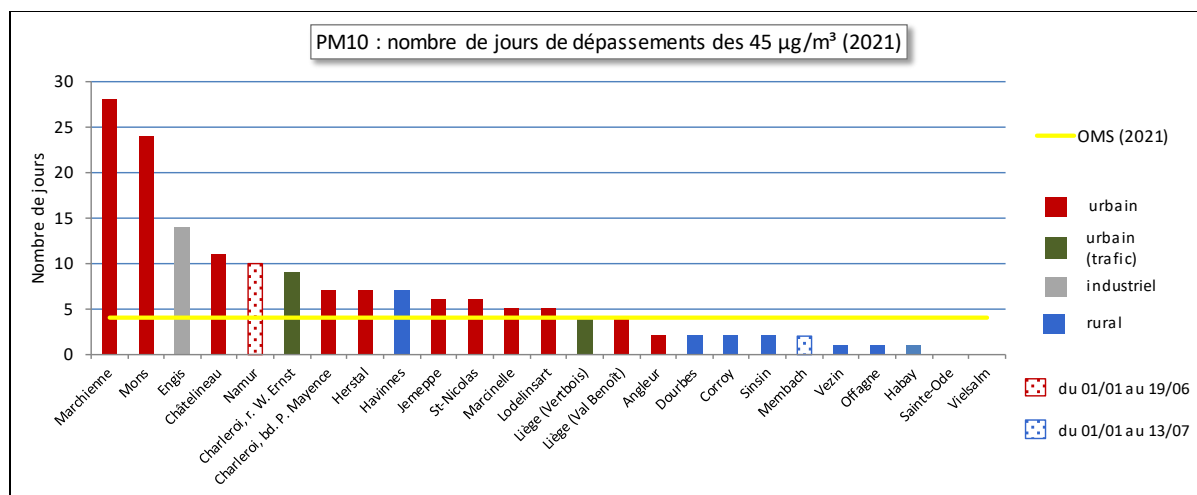
Figure 48 : PM10 - Classement des stations en fonction du nombre de dépassements journaliers (OMS-2021) – 2021
