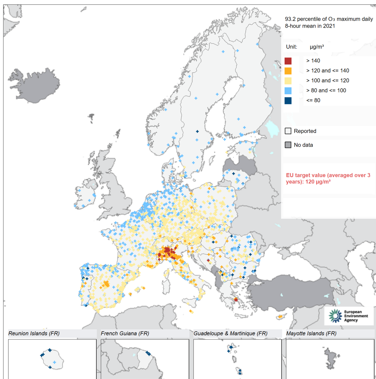
Figure 85 : Valeur cible européenne : la carte présente le percentile 93.2 du maximum journalier de la moyenne sur 8 h, correspondant au 26 ème maximum.
