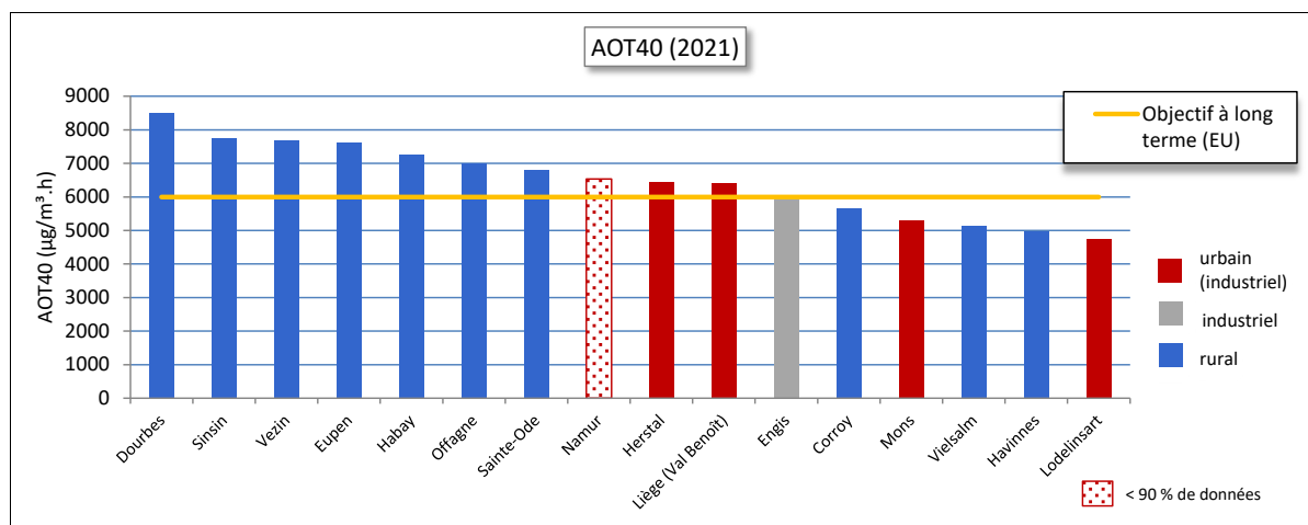
Figure 31 : AOT40 végétation – 2021
