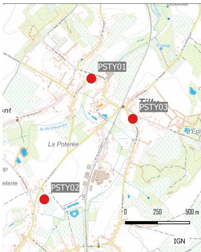
Figure 179 : Groupe de Tilly - Localisation des stations
