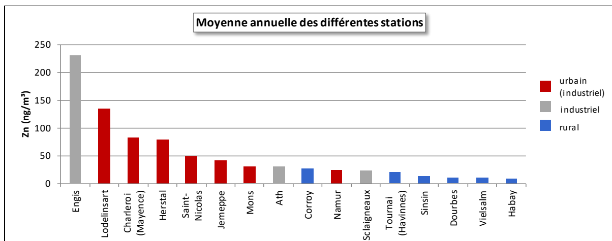
Figure 111 : Cadmium - Répartition des stations selon la moyenne annuelle en 2021
