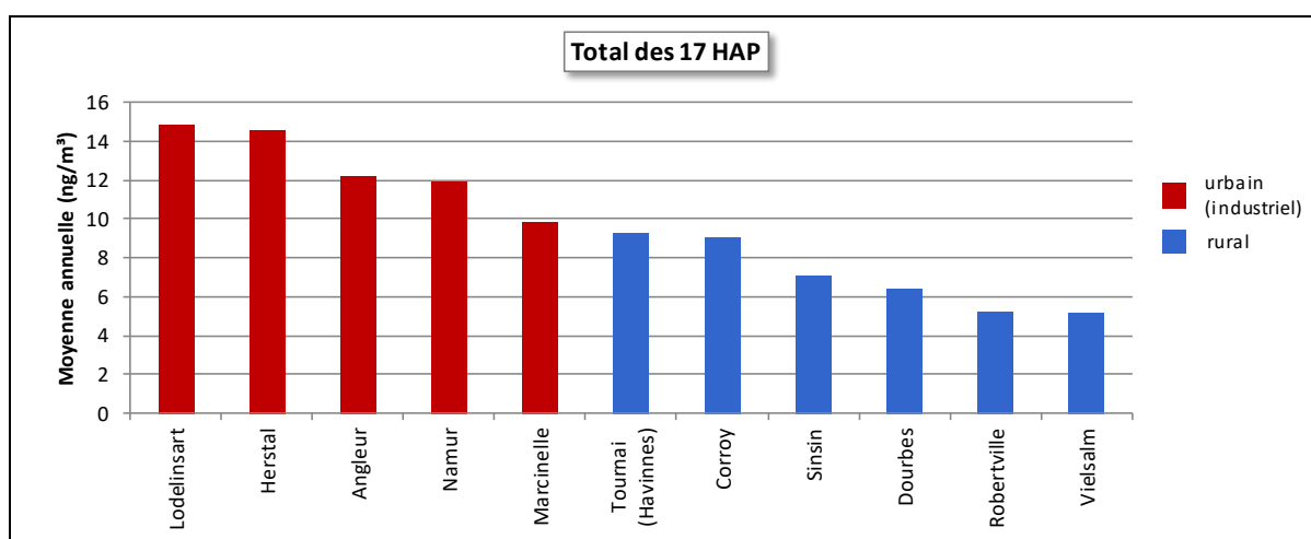
Figure 131 : Total des 17 HAP mesurés - Répartition des stations selon la moyenne annuelle en 2021
