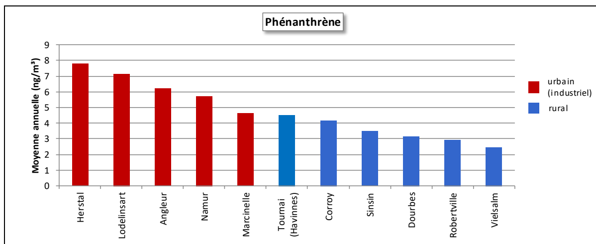
Figure 134 : Phénanthrène - Répartition des stations selon la moyenne annuelle en 2021
