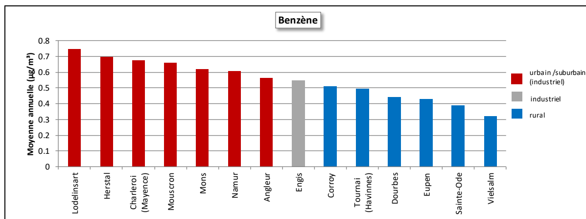
Figure 128 : Benzène - Répartition des stations selon la moyenne annuelle en 2021
