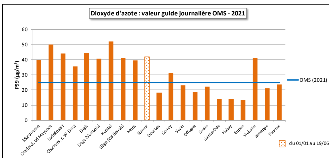
Figure 18 : Dioxyde d'azote – P99 des valeurs journalières et valeur guide en 2021
