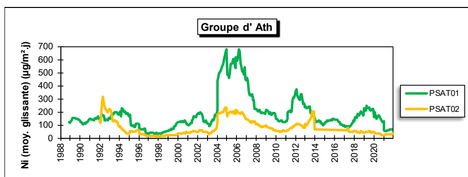
Figure 148 : Groupe d'Ath - Évolution à long terme des retombées en nickel
