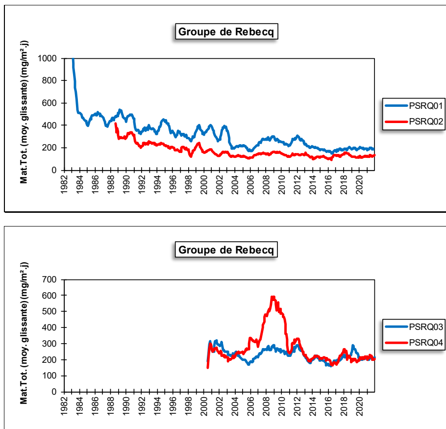
Figure 176 : Groupe de Rebecq - Évolution à long terme des retombées totales
