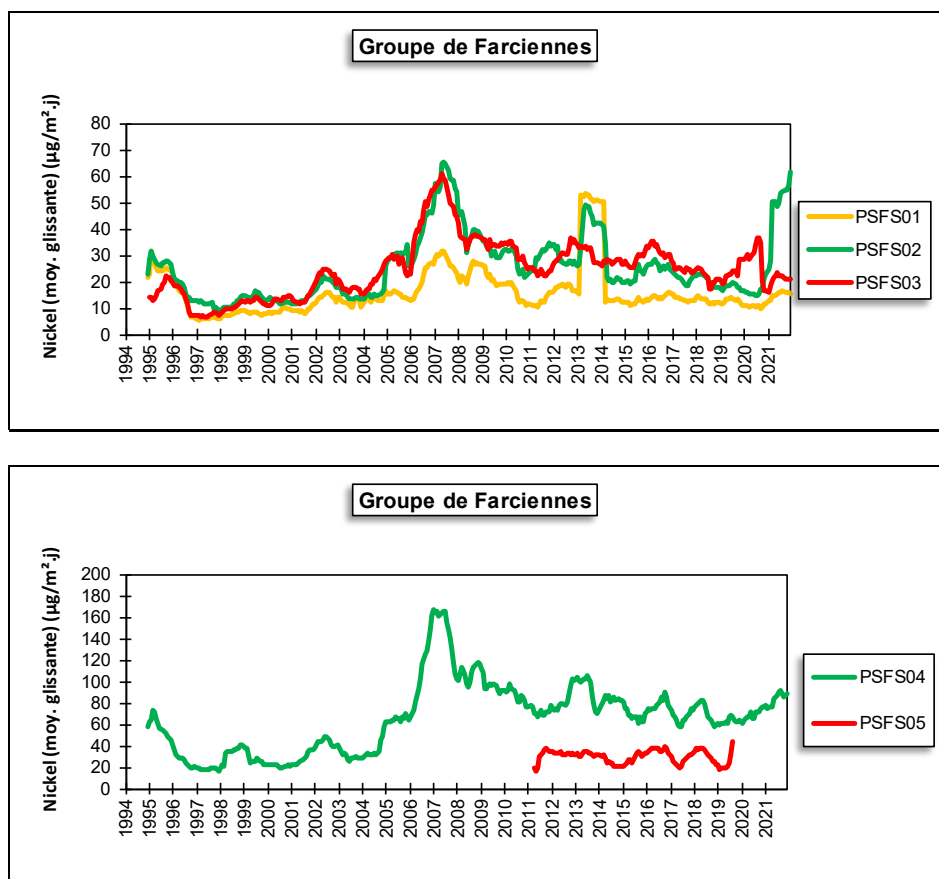
Figure 171 : Groupe de Farciennes - Évolution à long terme des retombées en nickel
