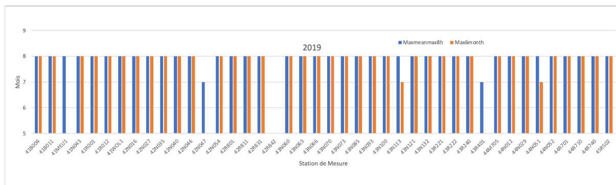
Figure 90 : Comparaison des périodes pour le maximum de la moyenne glissante sur 6 mois et du maximum de la moyenne glissante sur 6 mois des max 8h journaliers pour l'ensemble des stations de mesure, année 2019
